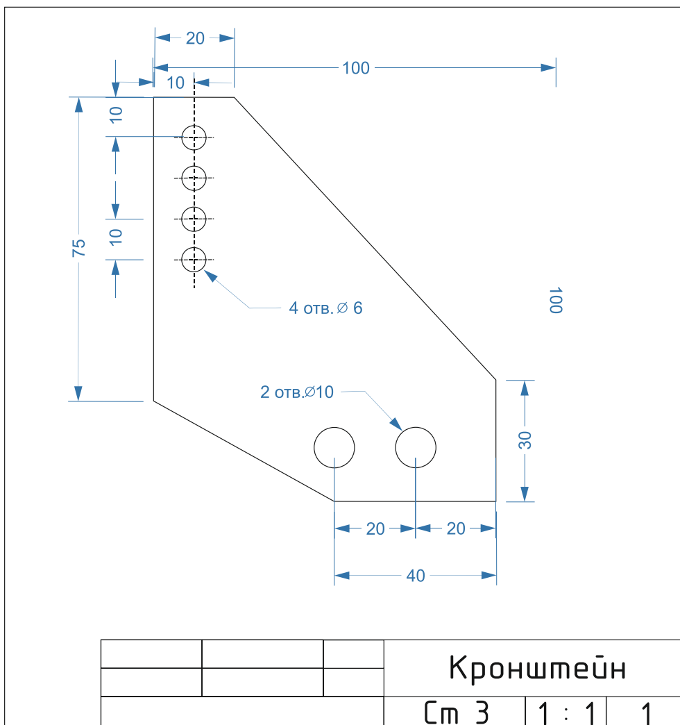
Рис. 1. Чертеж Кронштейн
